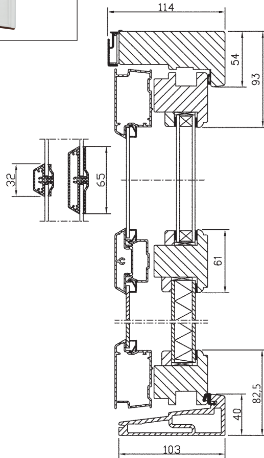
Vertikalsnitt
