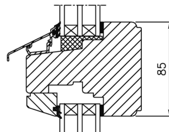
Vertikalsnitt karm tvärpost
