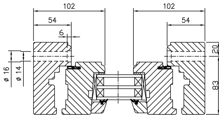
Horizontalsnitt
