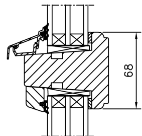
Liggande bågpost
