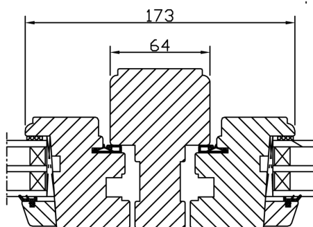
Horizontalsnitt karm mittpost
