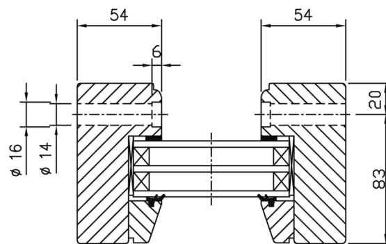
Horizontalsnitt
