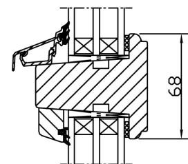
Liggande bågpost
