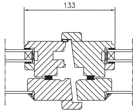
Horizontalsnitt pardörr
