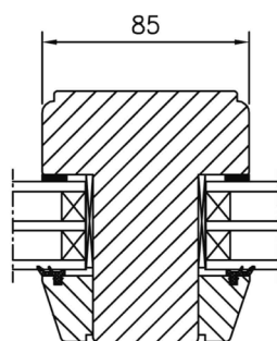
Horizontalsnitt karm tvärpost
