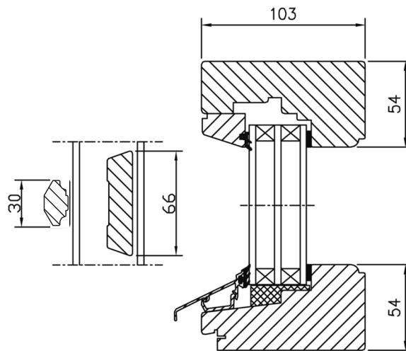
Vertikalsnitt
