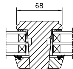
Stående bågpost
