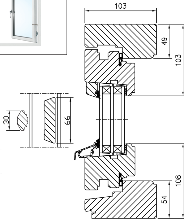
Vertikalsnitt
