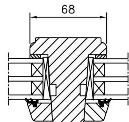
Stående bågpost
