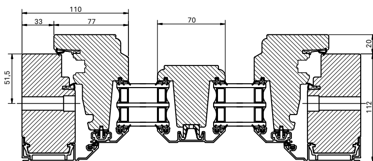
Horizontalsnitt
