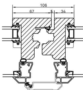
Horizontalsnitt pardörr
