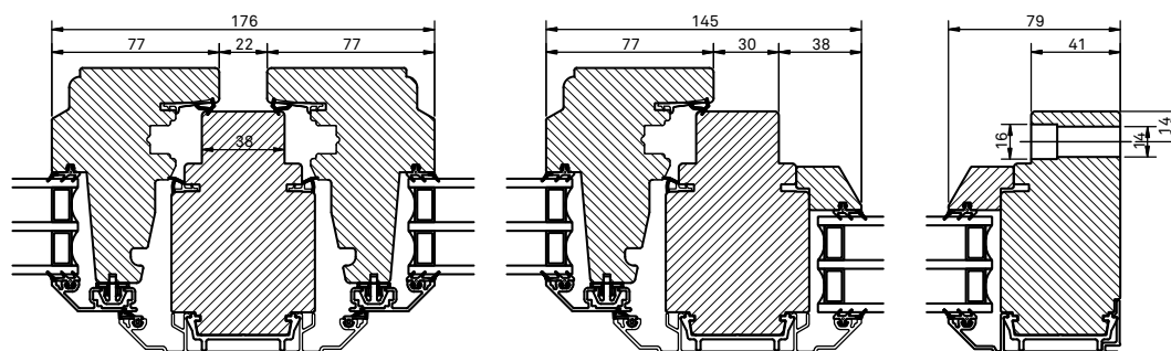
Horizontalsnitt karm mittpost
