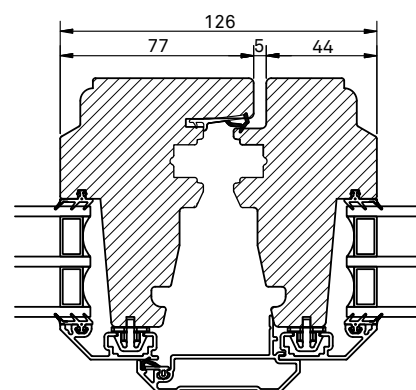
Horizontalsnitt pardörr
