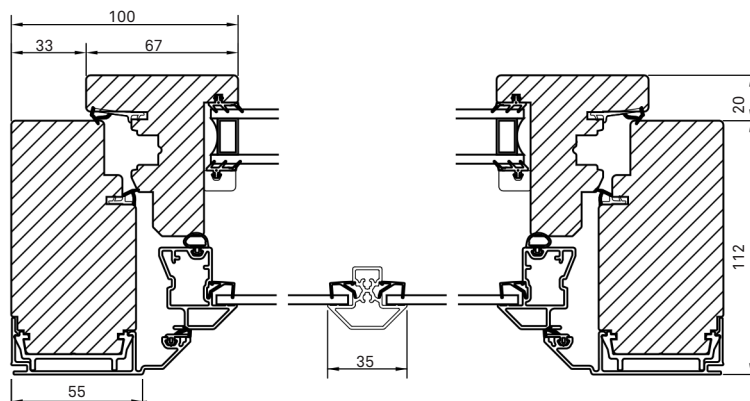
Horizontalsnitt
