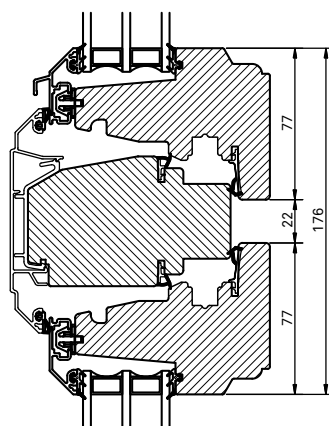
Vertikalsnitt karm tvärpost
