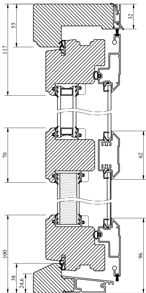
Vertikalsnitt
