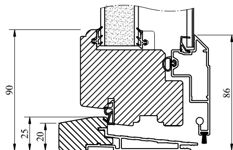
Alt. Tillval med Handikapptröskel
