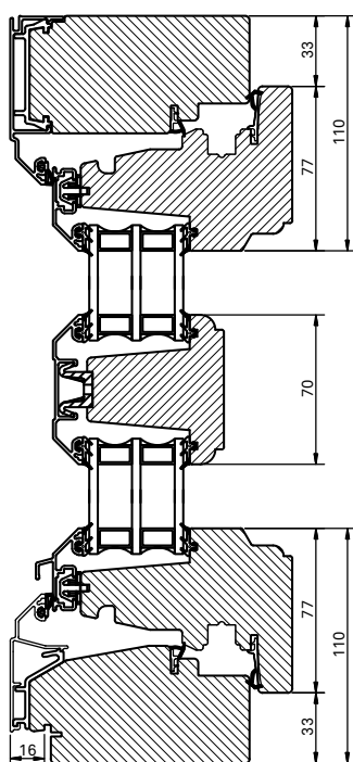
Vertikalsnitt
