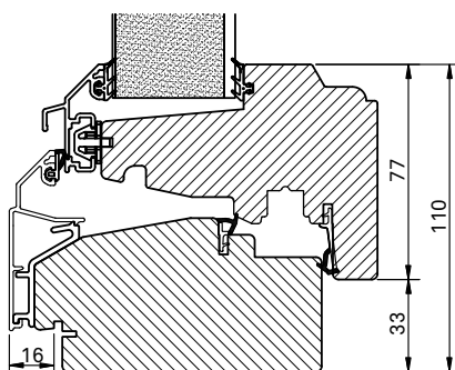
Vertikalsnitt
