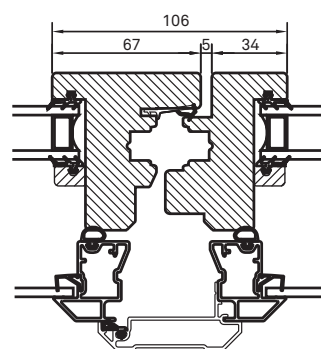
Horizontalsnitt mötesbåge
