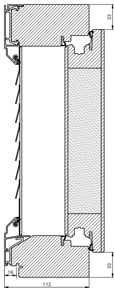
Vertikalsnitt
