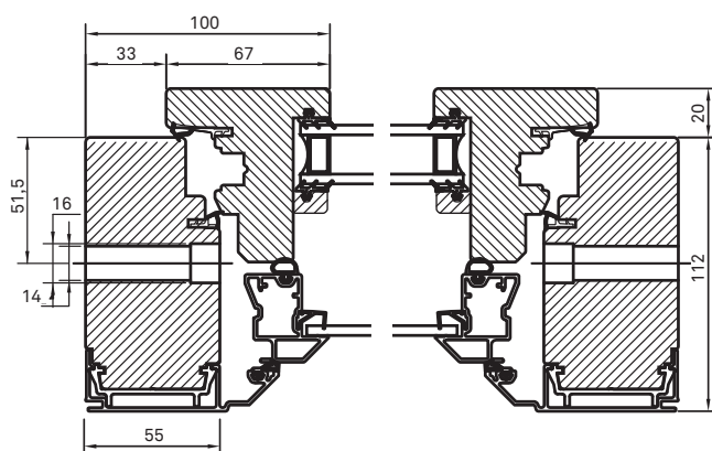
Horizontalsnitt
