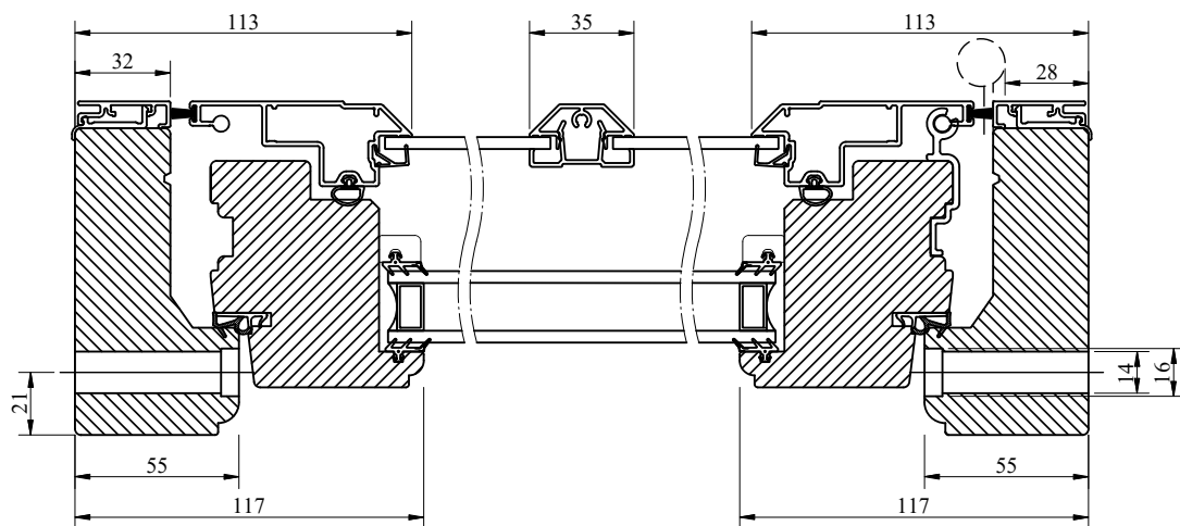
Horizontalsnitt
