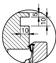
Spårfräsning insida
