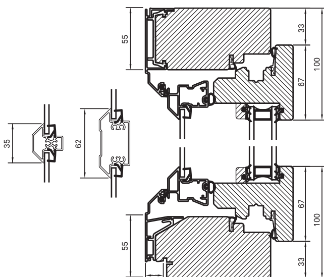
Vertikalsnitt
