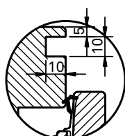
Spårfräsning insida
