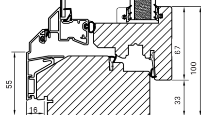
Vertikalsnitt
