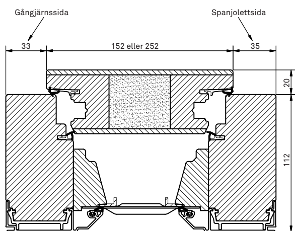
Horizontalsnitt
