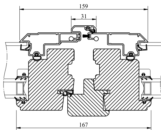
Horizontalsnitt pardörr
