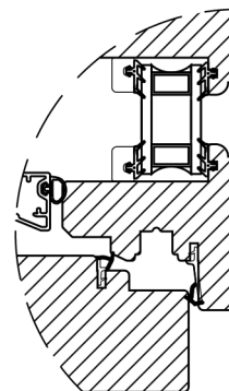
Profil insida
