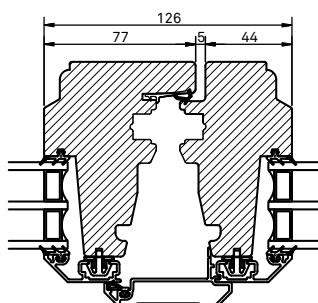
Horizontalsnitt mötesbåge
