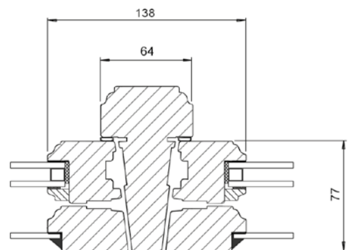
Horisontalsnitt karm mittpost
