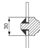
Vertikalsnitt spröjs standard
