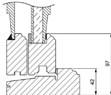
Vertikalsnitt
