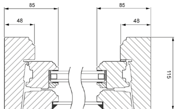
Horisontalsnitt
