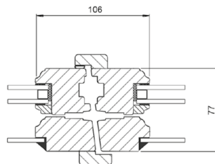
Horisontalsnitt mötesbåge
