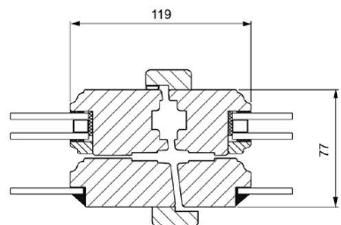
Horizontalsnitt pardörr
