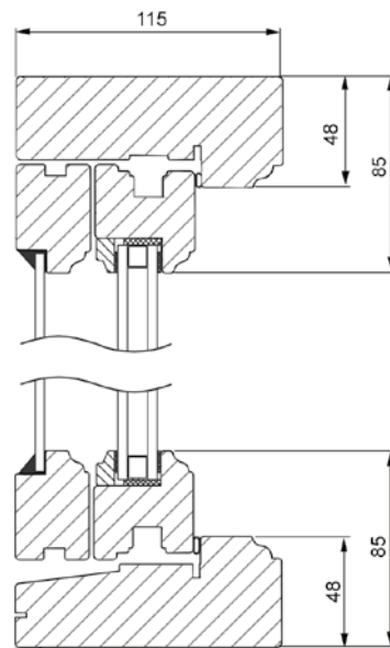
Vertikalsnitt
