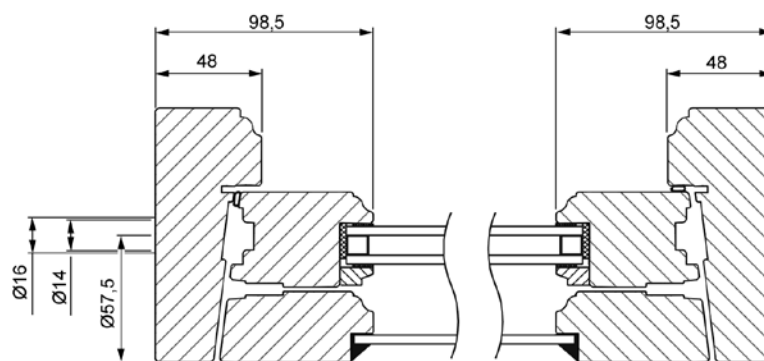
Horizontalsnitt
