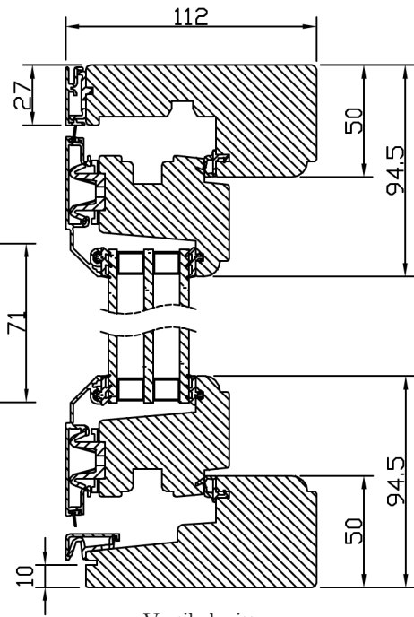
Vertikalsnitt
