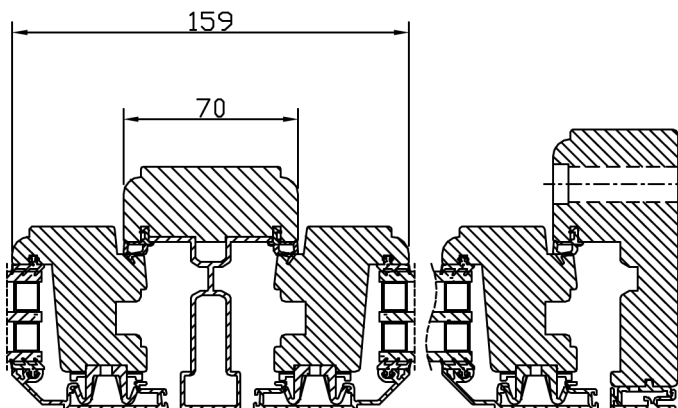
Horizontalsnitt karm mittpost
