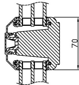
Vertikalsnitt bågpost
