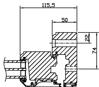
Horizontalsnitt
