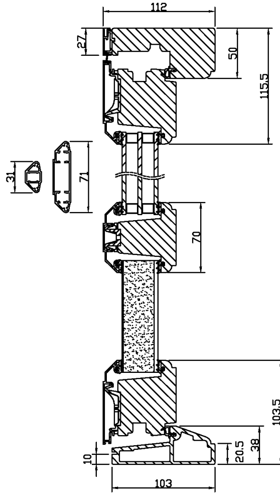
Vertikalsnitt
