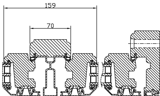
Horizontalsnitt karm mittpost
