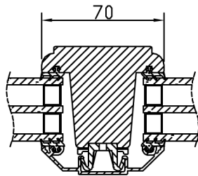
Horizontalsnitt bågpost
