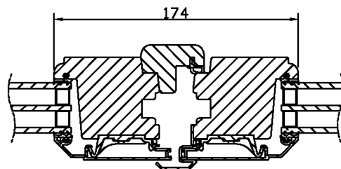
Horizontalsnitt pardörr
