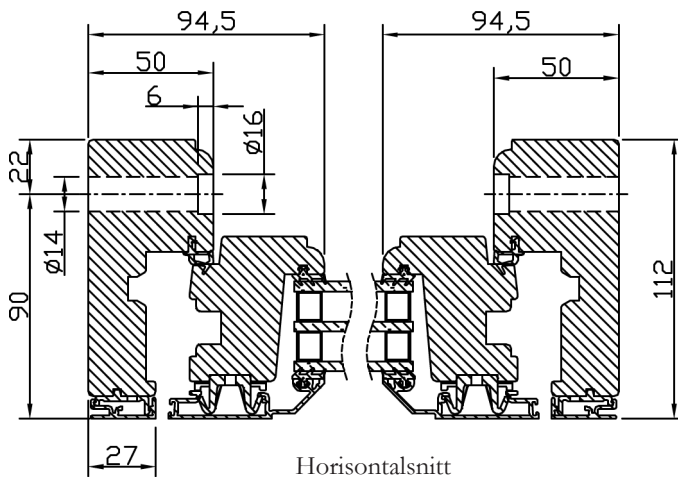
Horizontalsnitt bågpost
