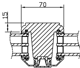
Horizontalsnitt karm mittpost
