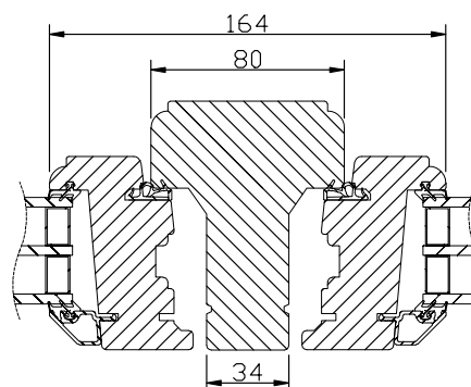
Horizontalsnitt karmpost
