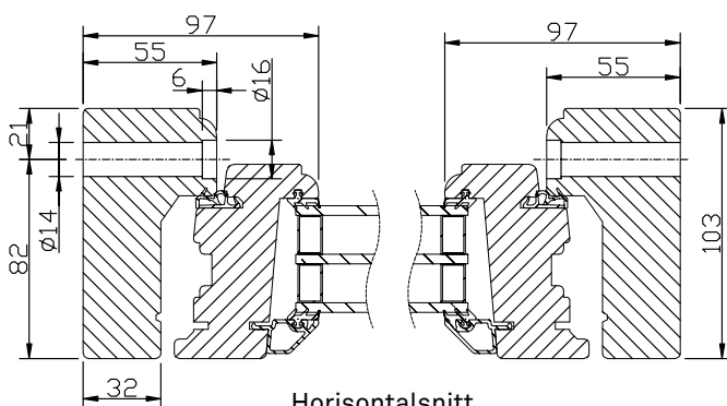
Horizontalsnitt
