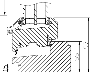
Vertikalsnitt
