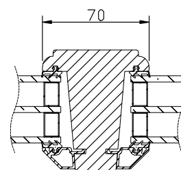
Horizontalsnitt bågpост
