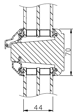
Vertikalsnitt bågpост
