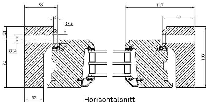
Horizontalsnitt
