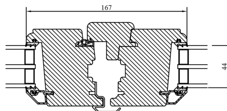
Horizontalsnitt Pardörr
