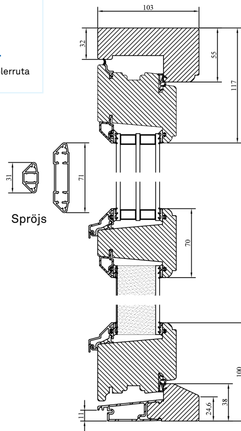
Vertikalsnitt
