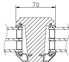
Horizontalsnitt bågpöst
