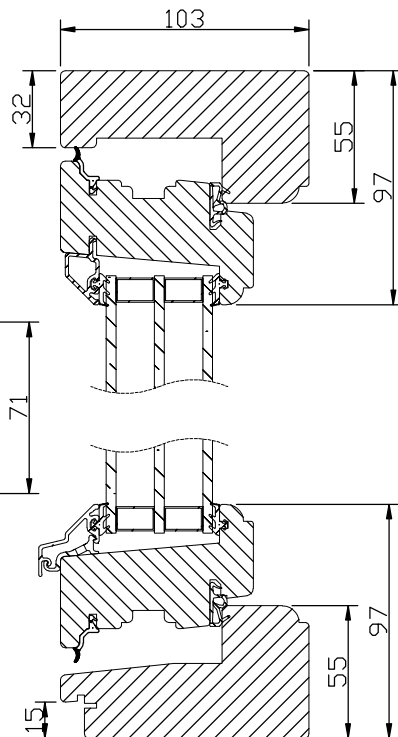
Vertikalsnitt
