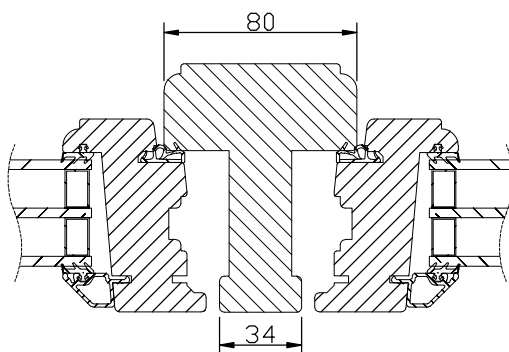
Horizontalsnitt karmpost
