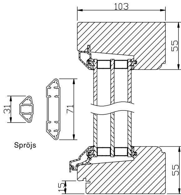
Vertikalsnitt
