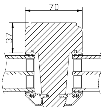
Horizontalsnitt karmpost
