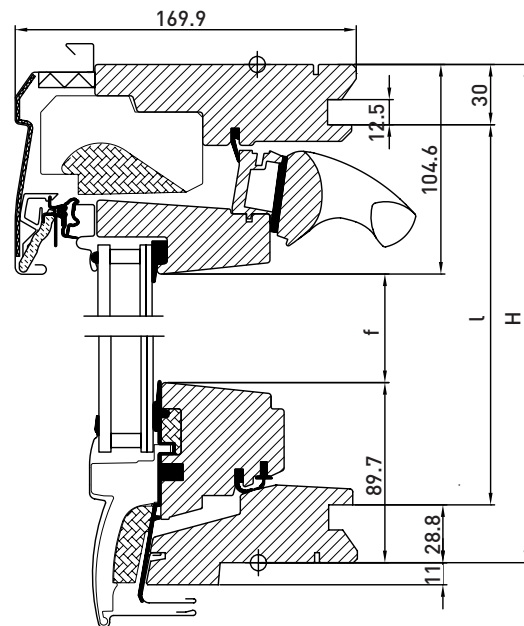
Vertikalsnitt
