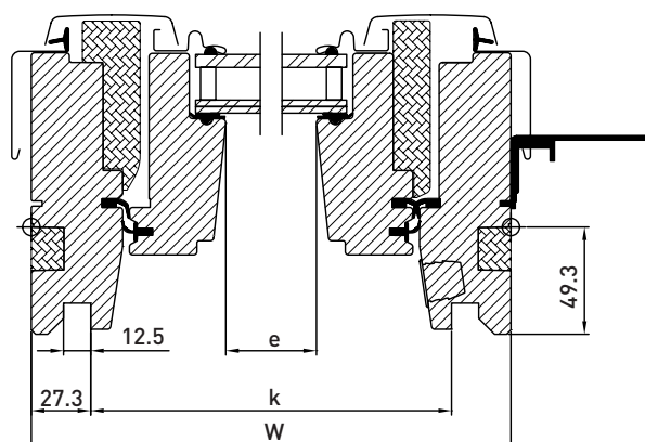
Horizontalsnitt
