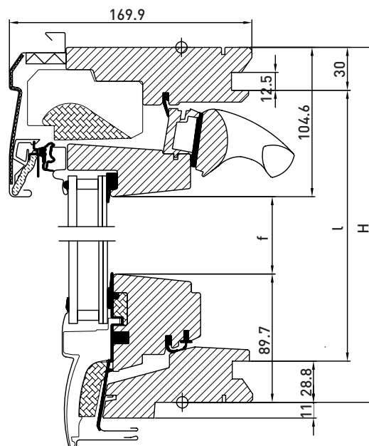
Vertikalsnitt
