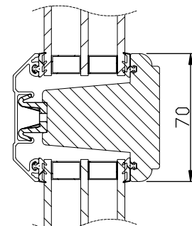
Vertikalsnitt bågpost
