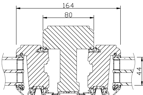
Horizontalsnitt karm mittpost
