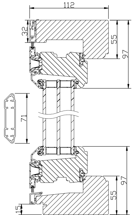
Vertikalsnitt
