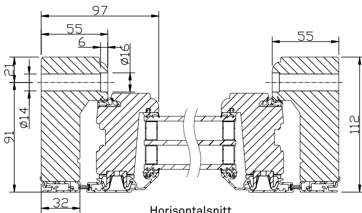
Horizontalsnitt
