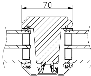
Horizontalsnitt bågpöst
