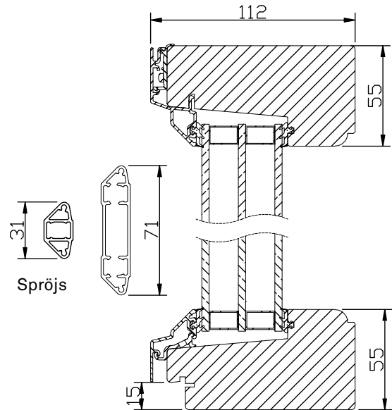
Vertikalsnitt
