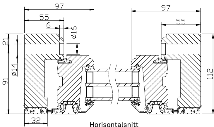
Horizontalsnitt
