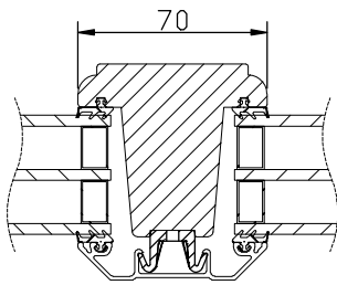
Horizontalsnitt bågpost
