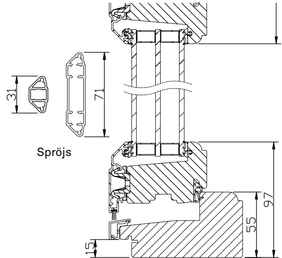
Vertikalsnitt
