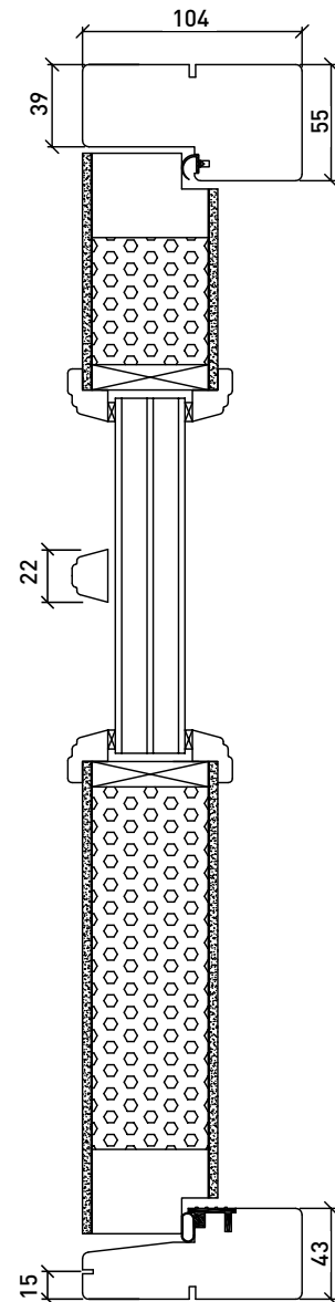
Vertikalsnitt
