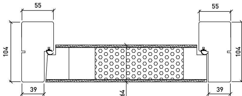
Horizontalsnitt
