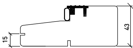
Standardtröskel
