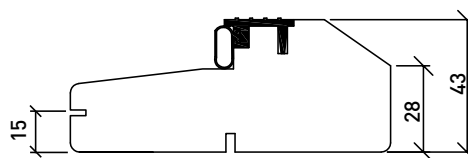
Fasad tröskel
