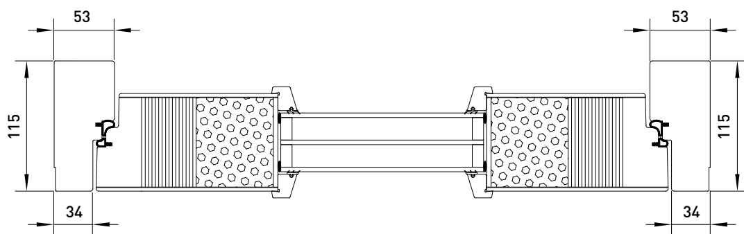
Horizontalsnitt
