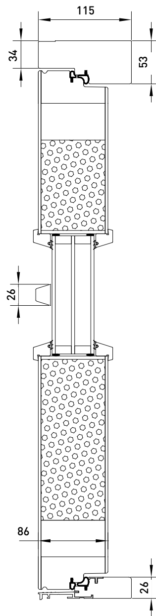
Vertikalsnitt
